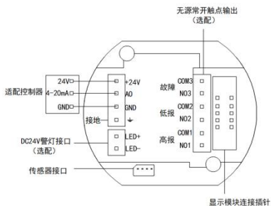
图 4-2 接线示意图
